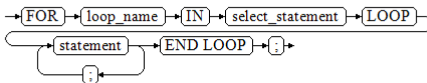
图 10-34 FOR_AS_loop::=
